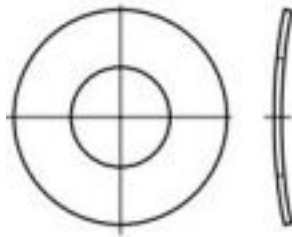
Podkładki podatne łukowe i faliste DIN 137/ PN-82037 i PN-82038
