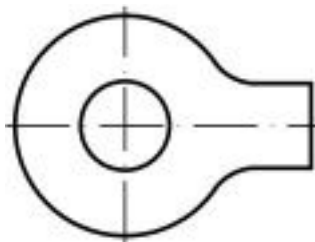
Podkładki odginane jednołapkowe DIN93/ PN-82021
