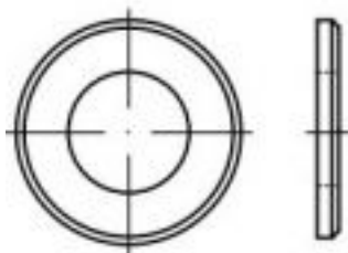
Podkładki okrągłe DIN 125 i DIN 126/ PN-82005 i PN 82006/ ISO 7089,7090,7091
