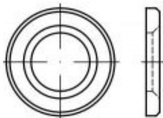
Podkładki okrągłe do połączeń sprężanych HV EN 14399-6/ DIN 6916/ PN-82039
